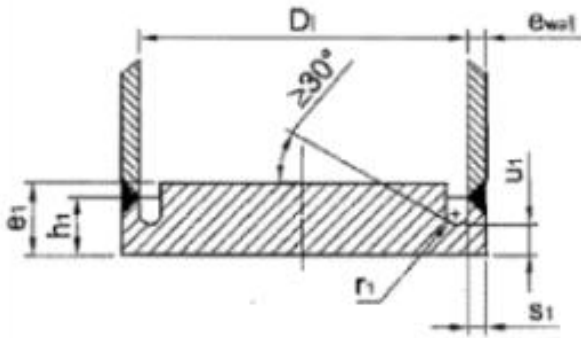
[ 그림 XI.2 - 릴리빙 홈을 가진 편평한 기초 ]
